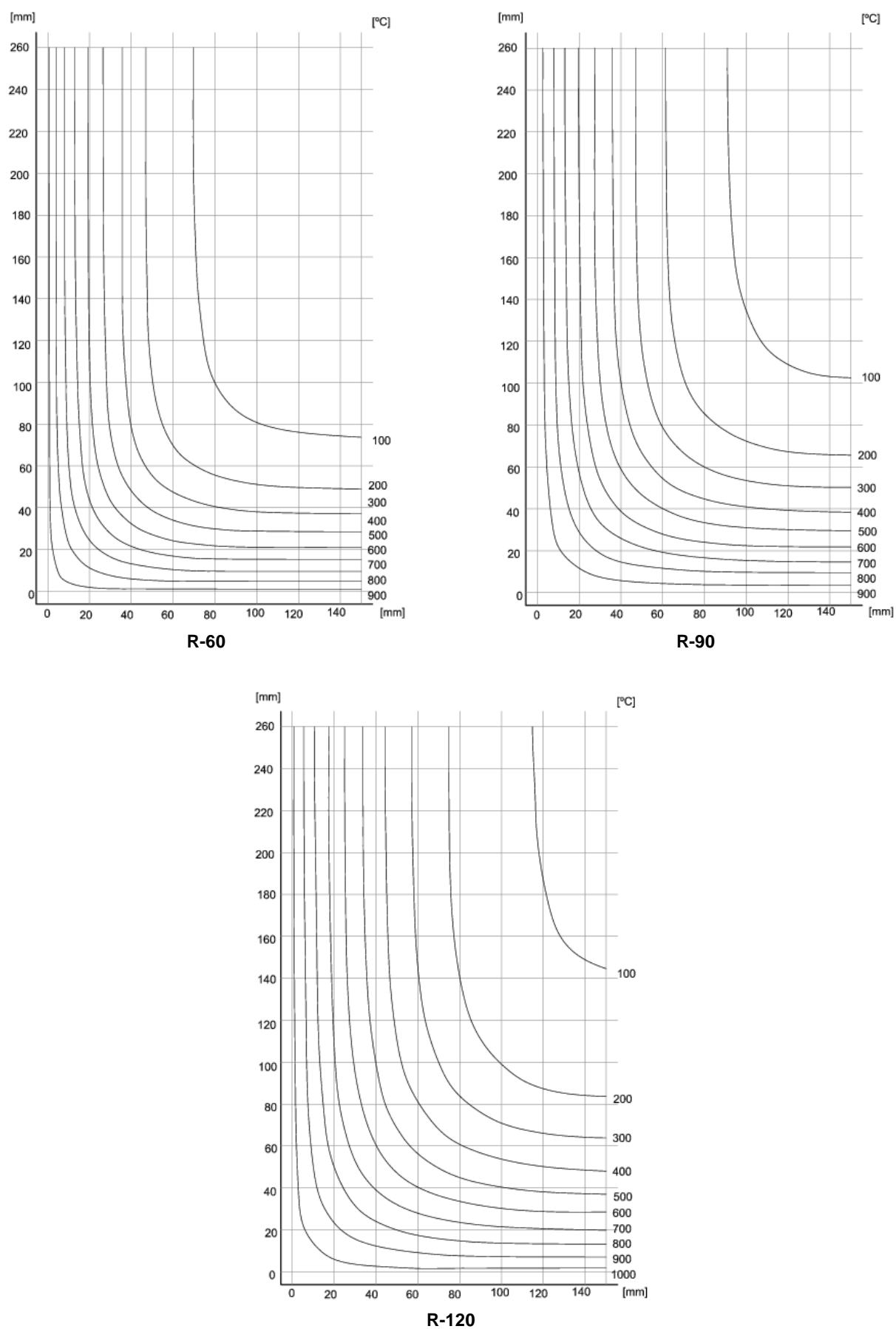
Figura C.4. Isothermas para cuartos de sección de 600 x 300 mm expuestos por ambas caras
